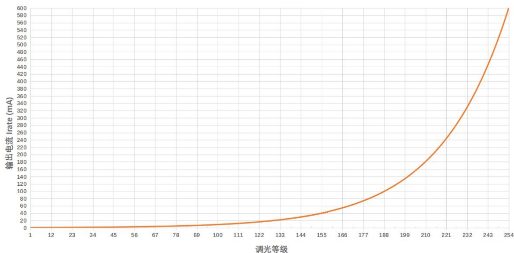
DALI调光曲线图
